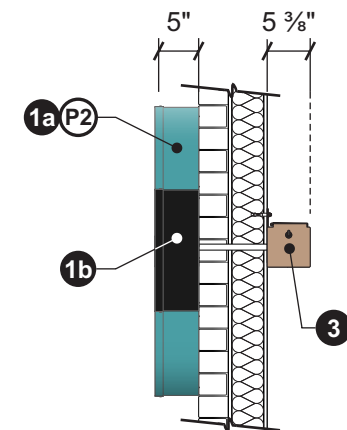
2 END VIEW 1.0 SCALE: 1/2" = 1'-0"
