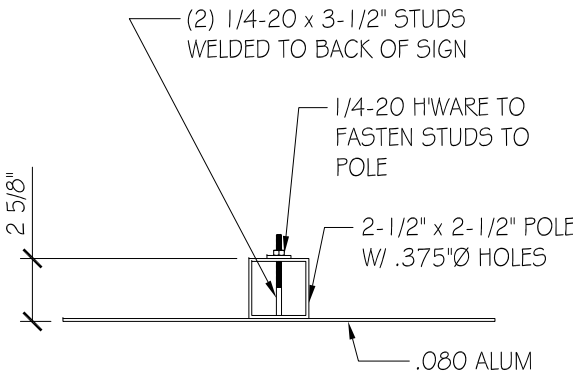
PLAN VIEW SCALE: 1-1/2" = 1'-0"
