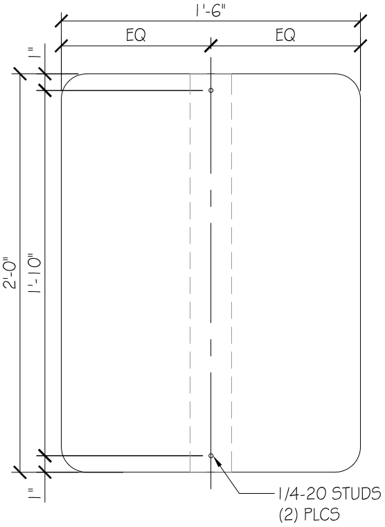
REAR DETAIL SCALE: 1-1/2" = 1'-0"
