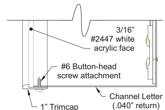
4 ENLARGED END SECTION 1.0 SCALE: N.T.S.
