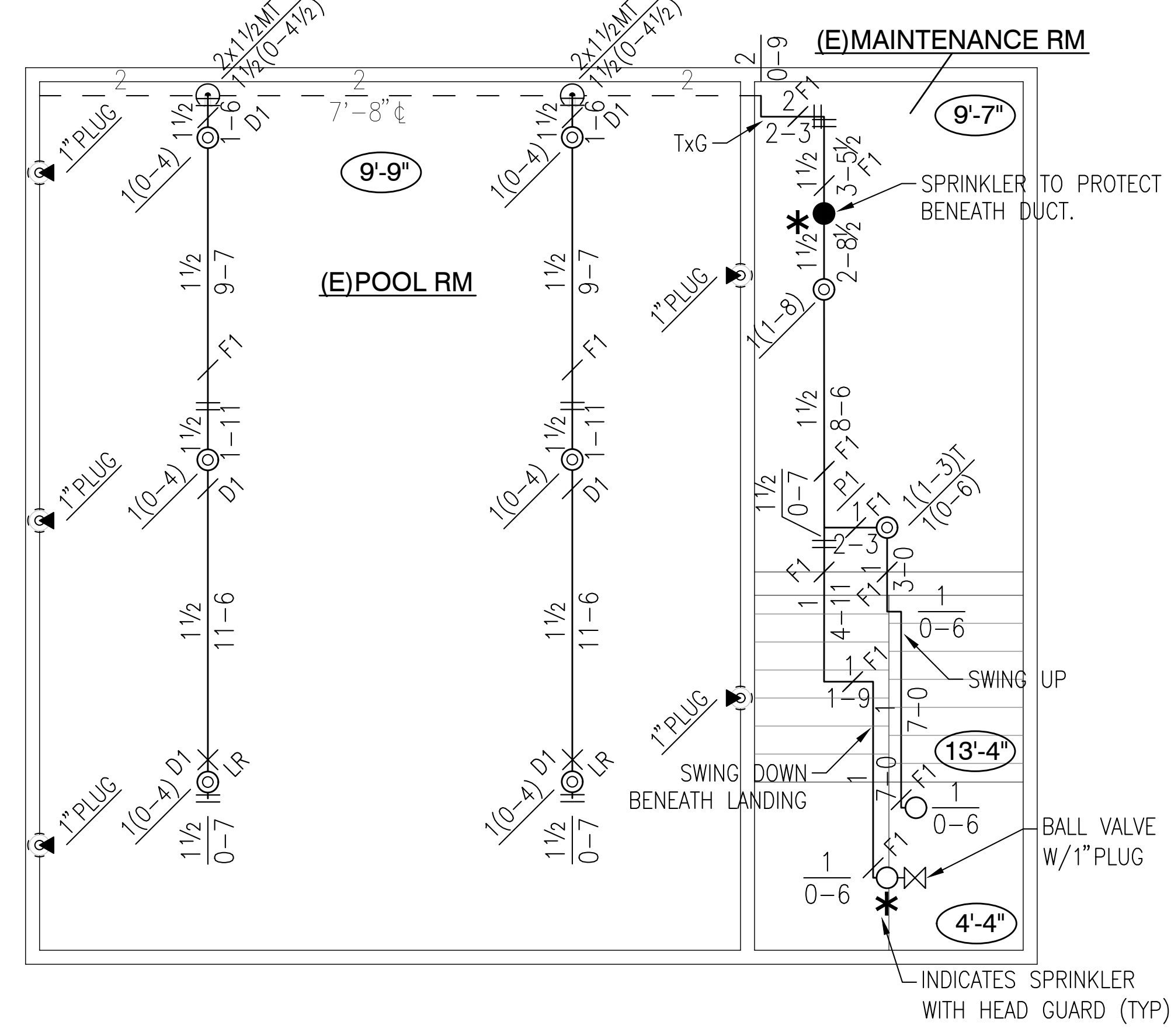
FIRE SPRINKLER PLAN SCALE: 1/8"=1'-0"
