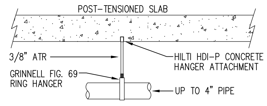
F1 HANGER DETAIL SCALE: NONE
