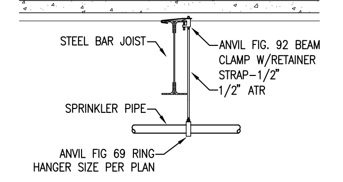
D1 HANGER DETAIL SCALE: NONE
