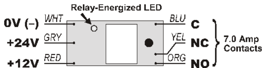
PAM-2
