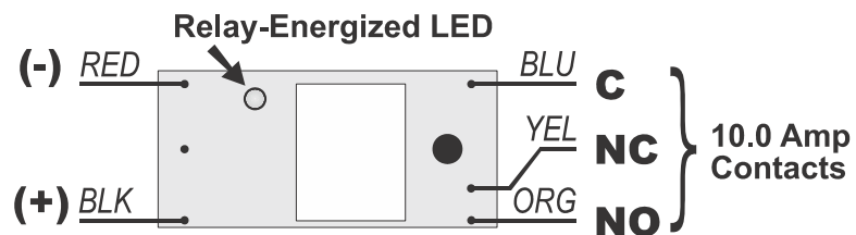
PAM-4
