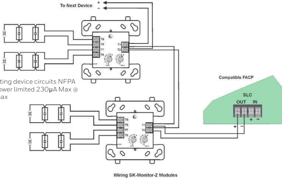
Wiring SK-Monitor-2 Modules
