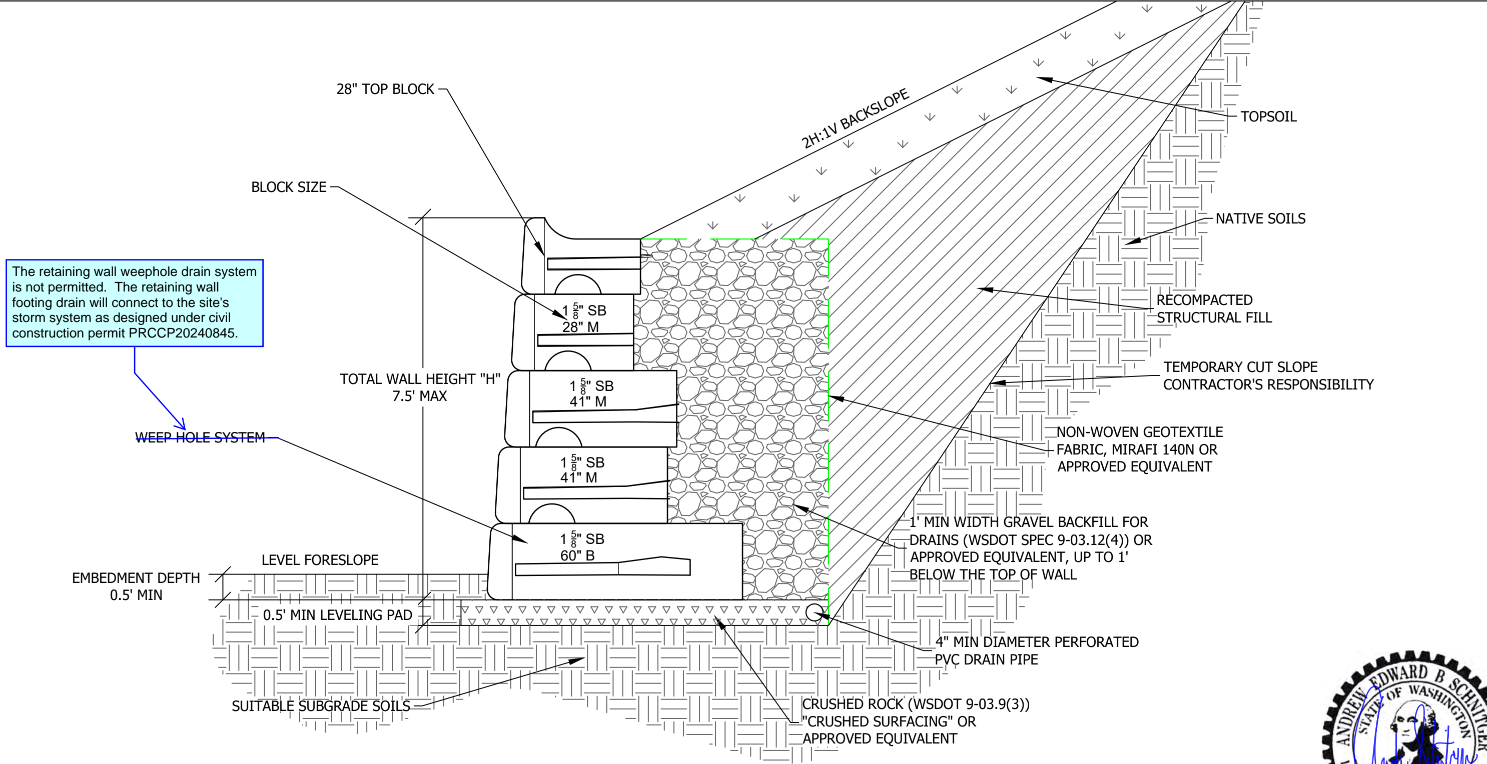
WALL B (NO SCALE)
