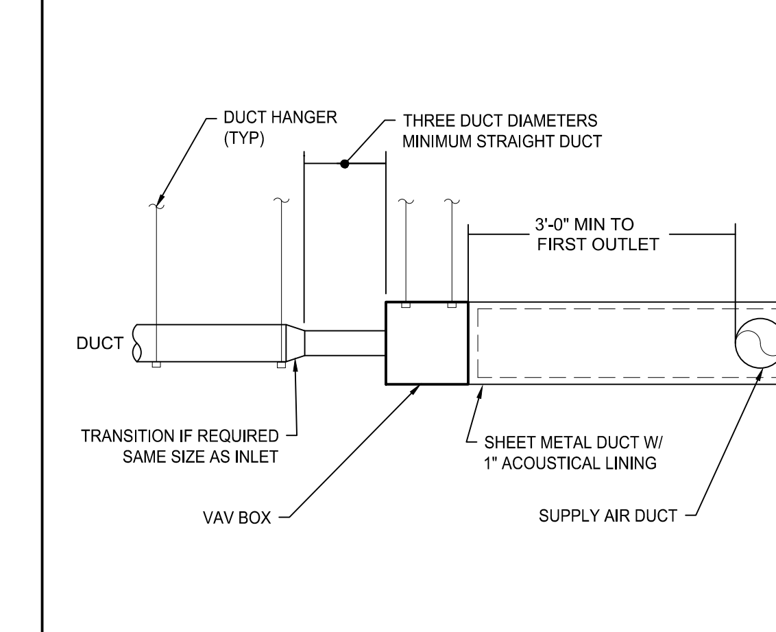
4 TM6.01 VAV BOX DETAIL N.T.S.
