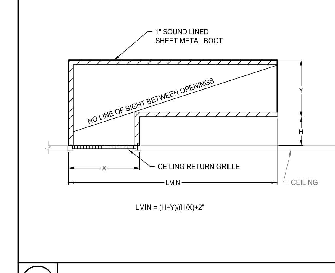
1 TM6.01 RETURN AIR BOOT DETAIL N.T.S.
