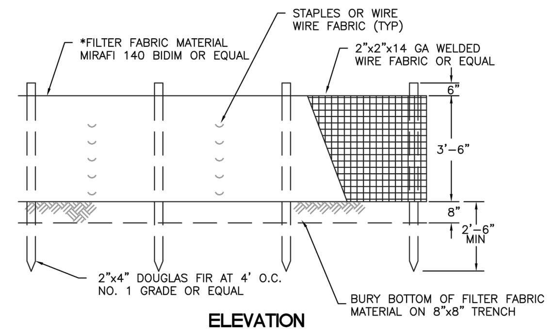
ELEVATION
