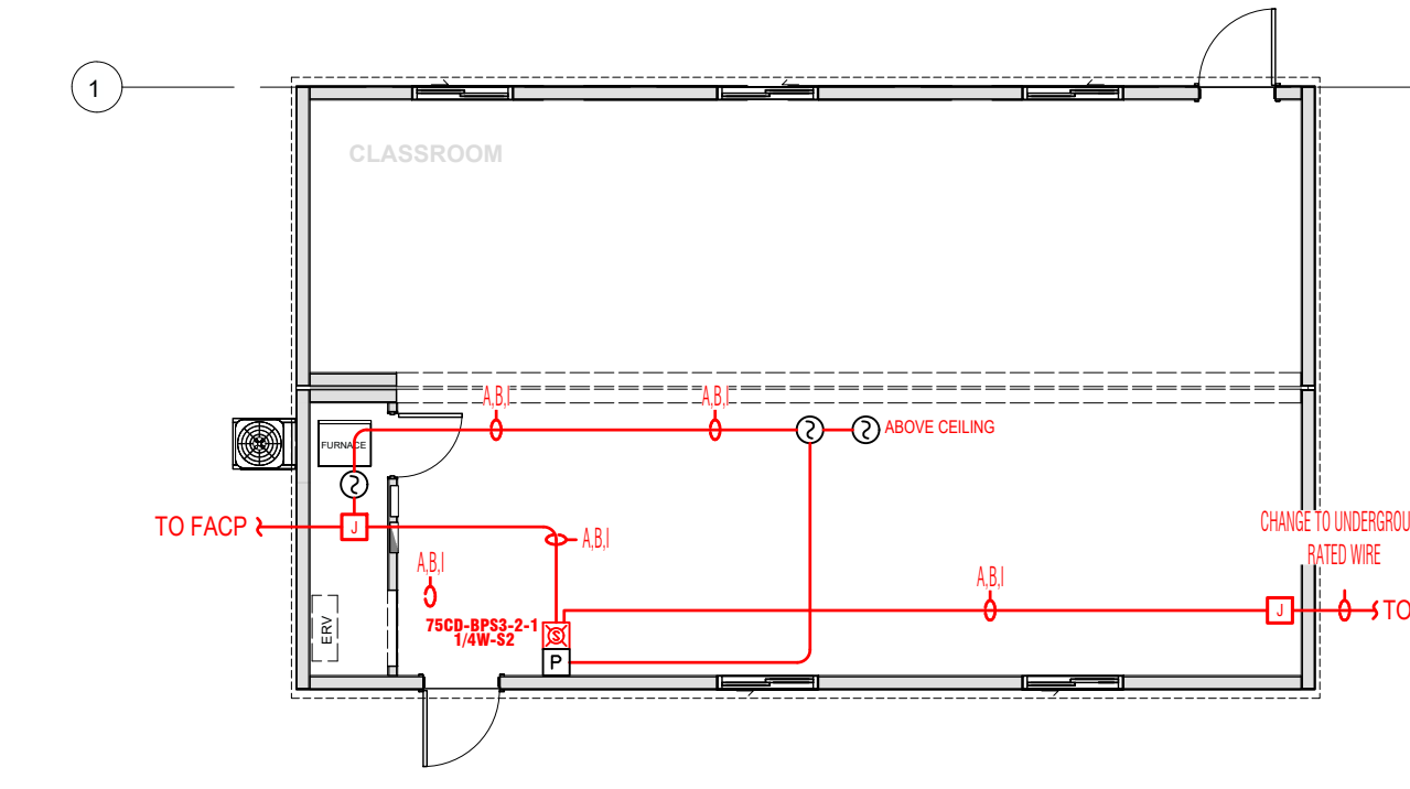
PORTABLE 11 SCALE: 1/8" = 1'-0"
