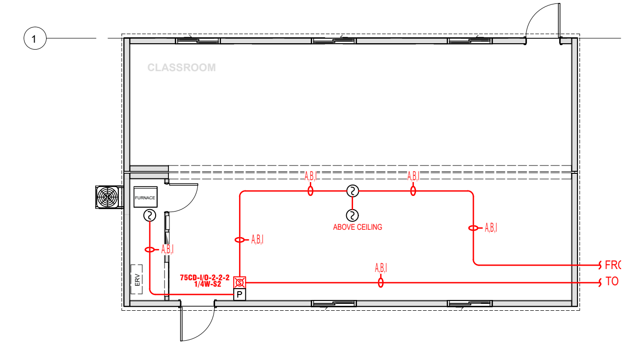
PORTABLE 8 SCALE: 1/8" = 1'-0"
