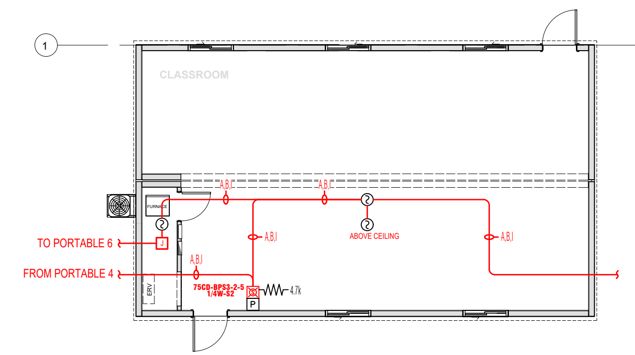
PORTABLE 5 SCALE: 1/8" = 1'-0"
