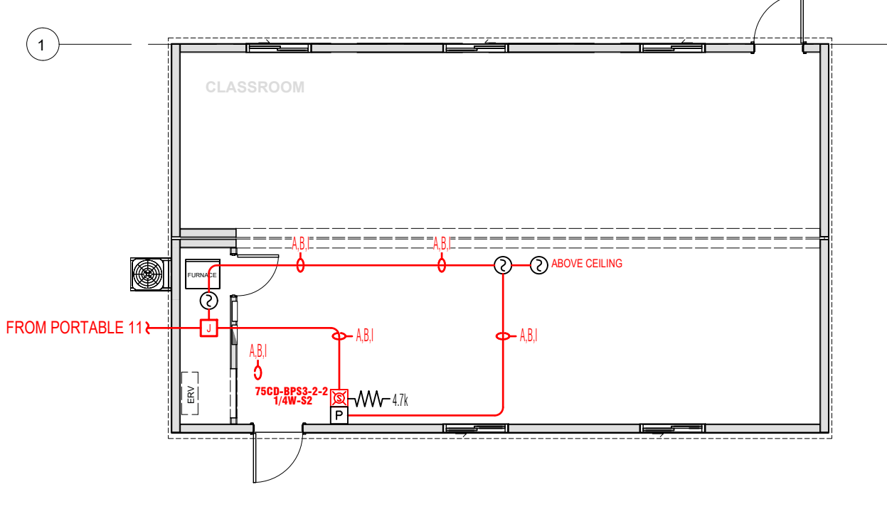
PORTABLE 12 SCALE: 1/8" = 1'-0"
