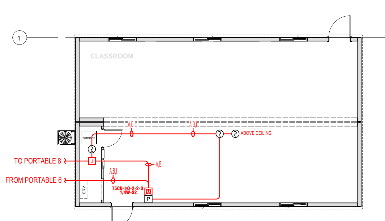
PORTABLE 7 SCALE: 1/8" = 1'-0"
