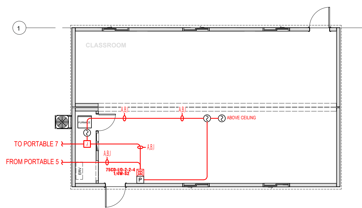
PORTABLE 6 SCALE: 1/8" = 1'-0"
