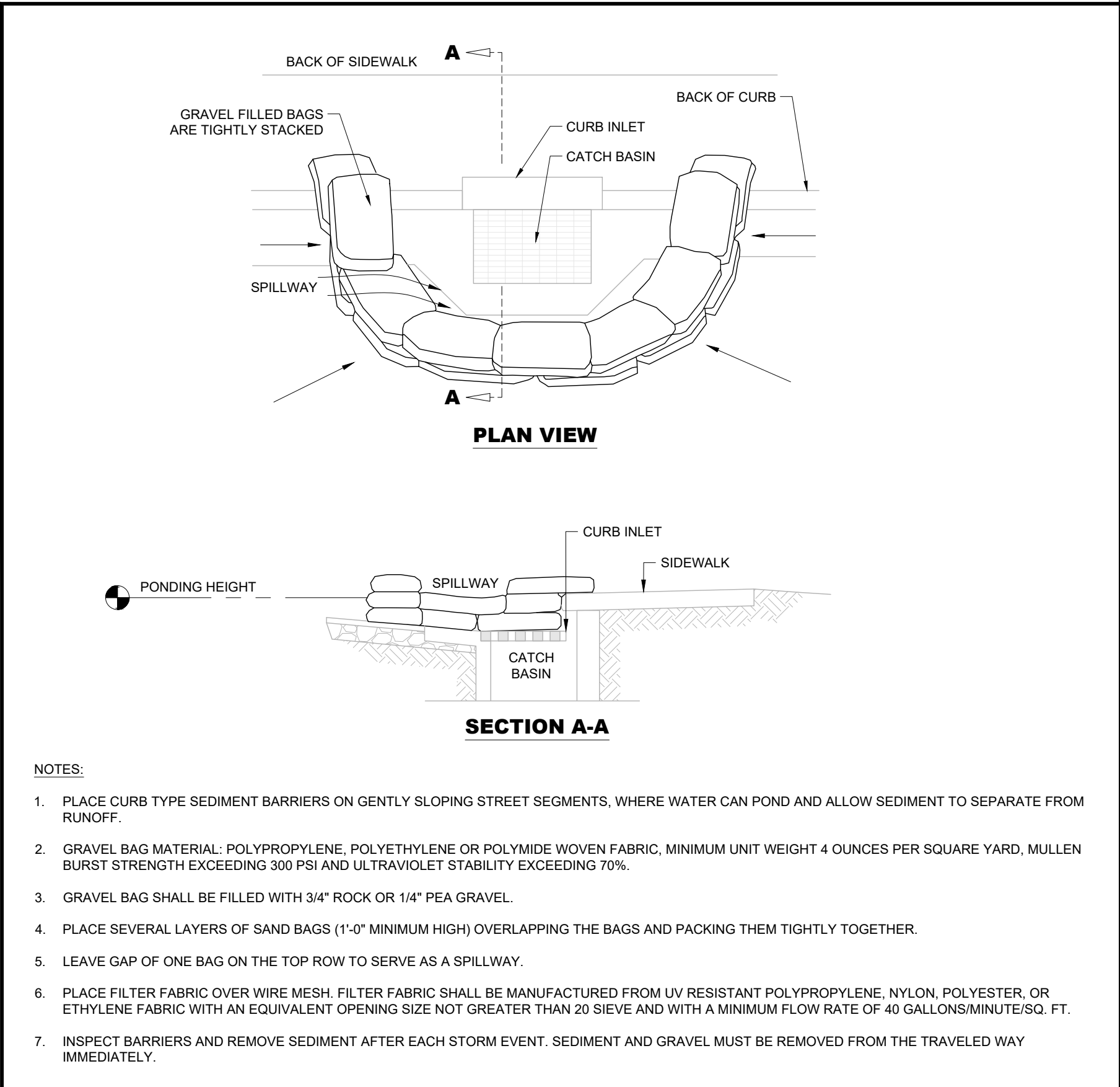
CURB INLET SEDIMENT BARRIER SCALE N.T.S. 1
