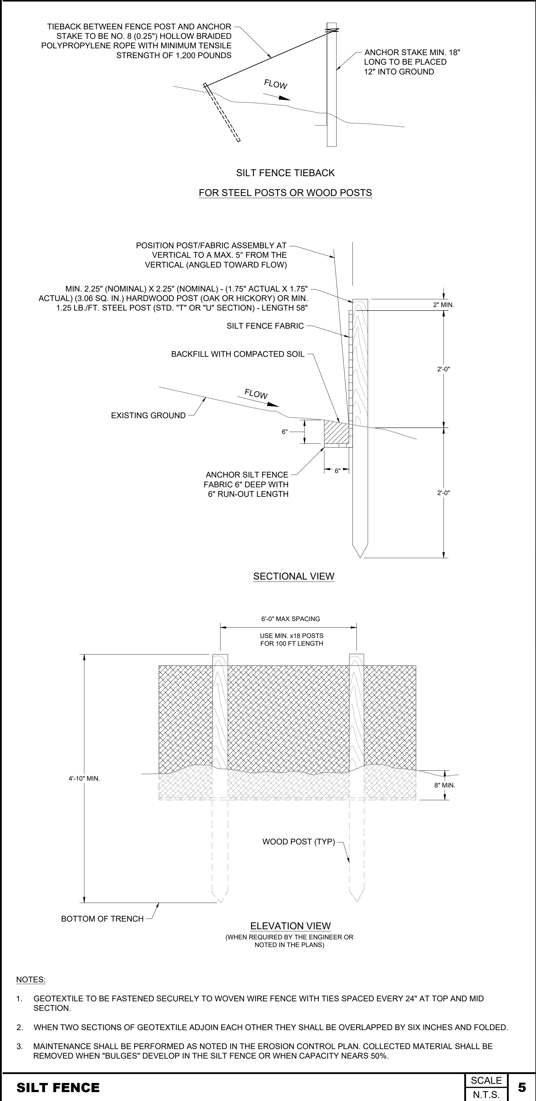
SILT FENCE SCALE N.T.S. 5
