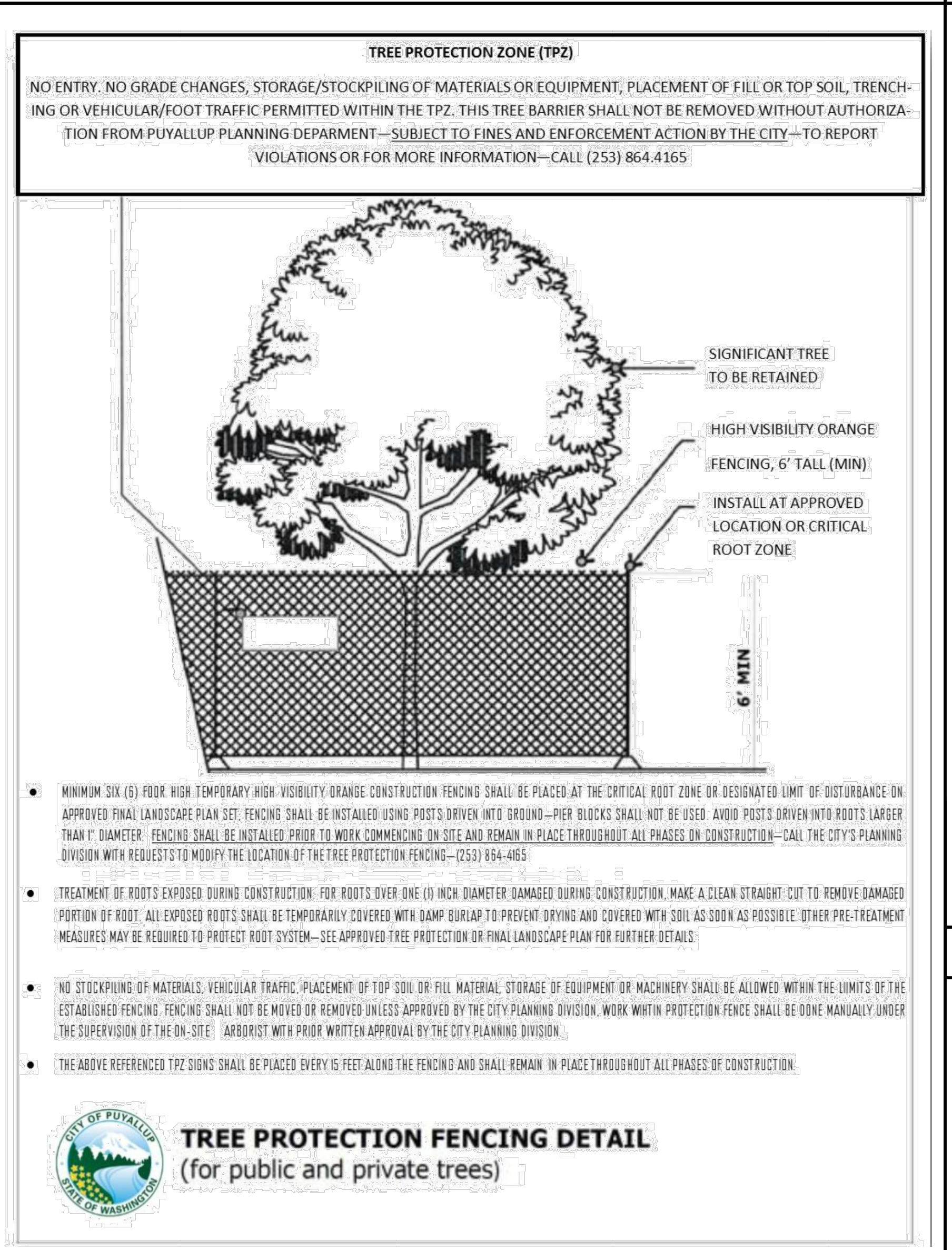
TREE PROTECTION SCALE N.T.S. 3
