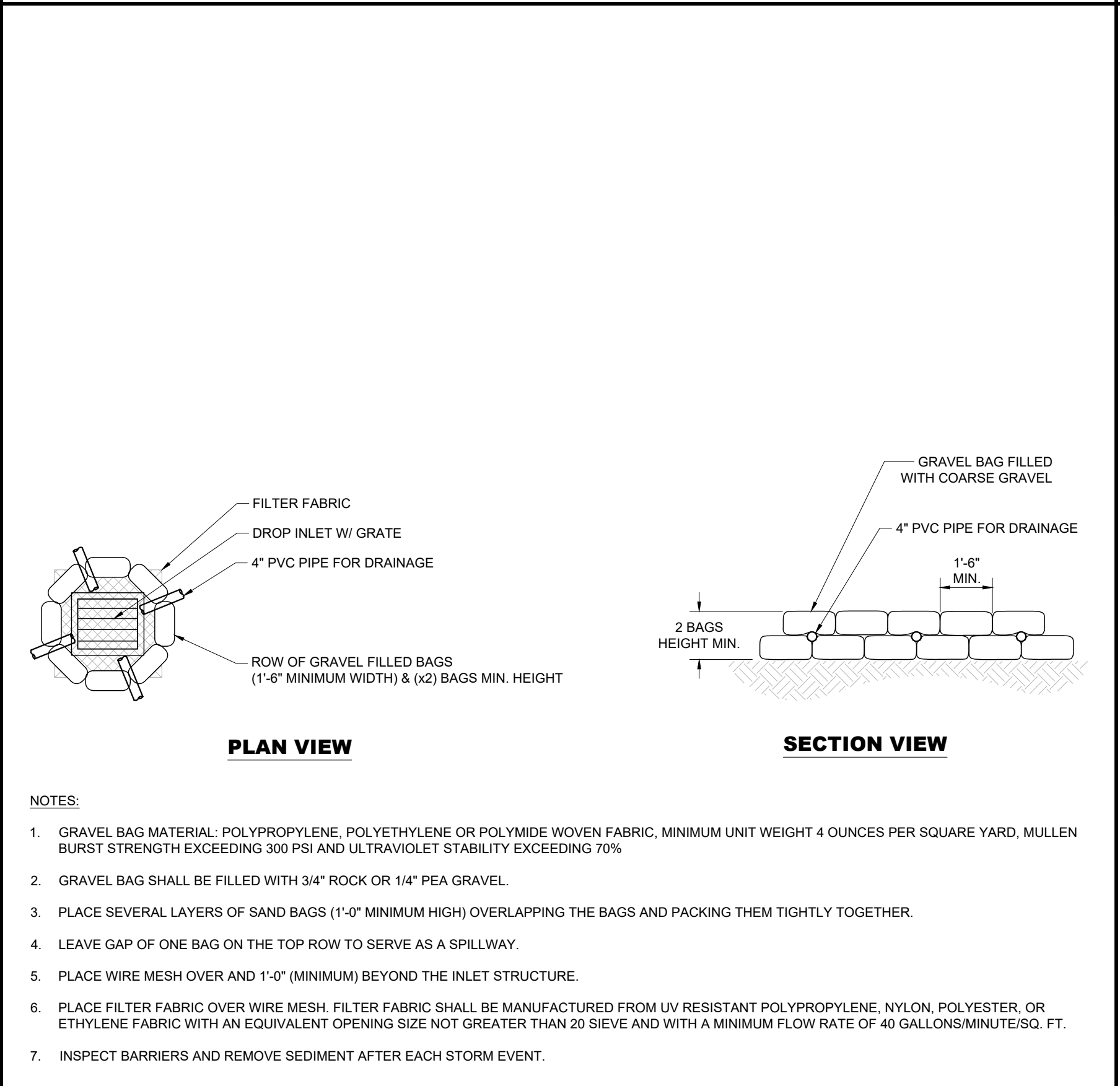
DROP INLET SEDIMENT BARRIER SCALE N.T.S. 2
